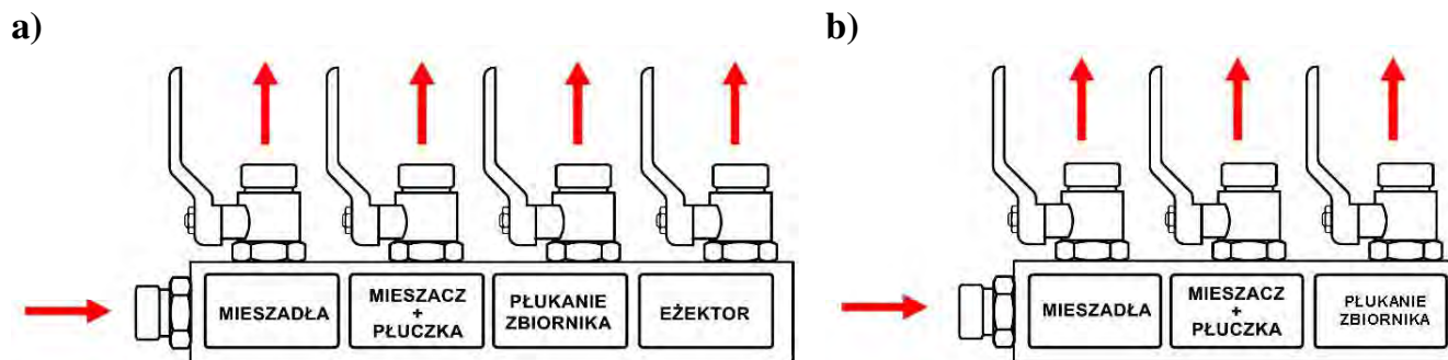
Rys. 17. Listwa zaworów (kolektor zaworów)- schemat
