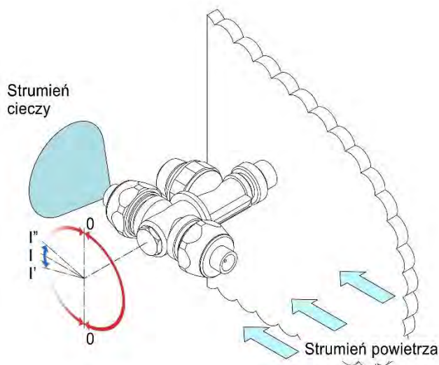
Rys. 33. Schemat nastawień korpusów rozpylaczy
