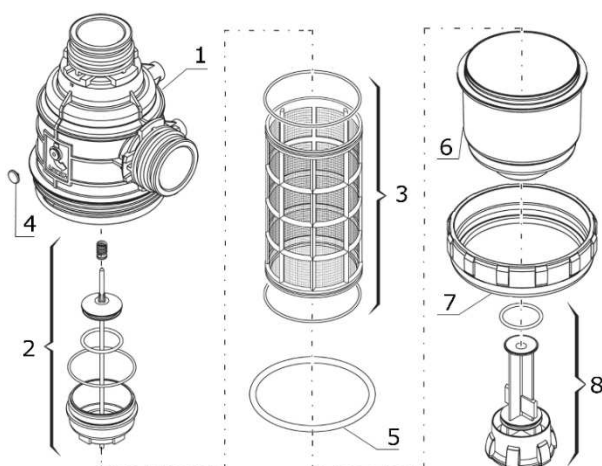
Rys. 27. Filtr ssawny. a) schemat; b) widok
