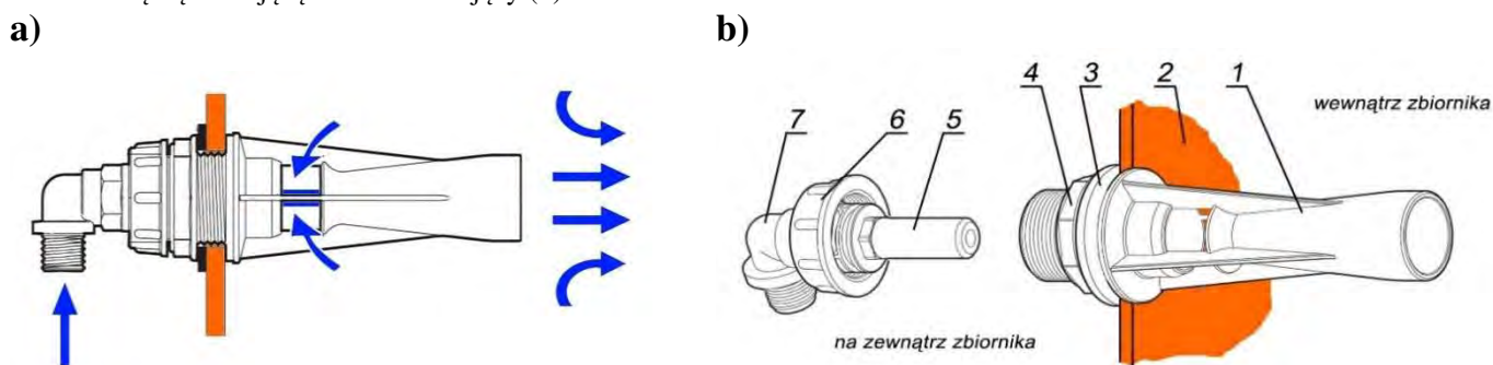
Rys. 18. Mieszadło hydrauliczne:
