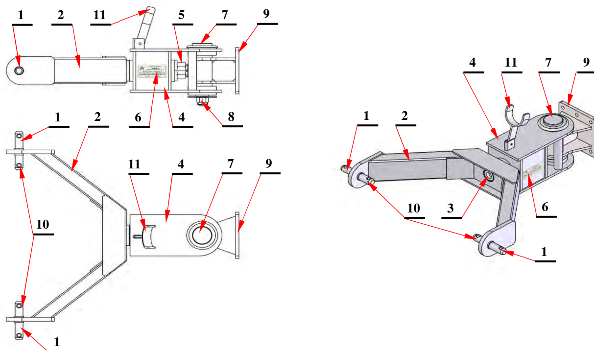
Rys. 48. Schemat zaczepu skrętnego kategorii 2N
