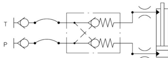
Rys. 45. Schemat hydrauliczny podłączenie cylindra hydraulicznego kierownic powietrza.
