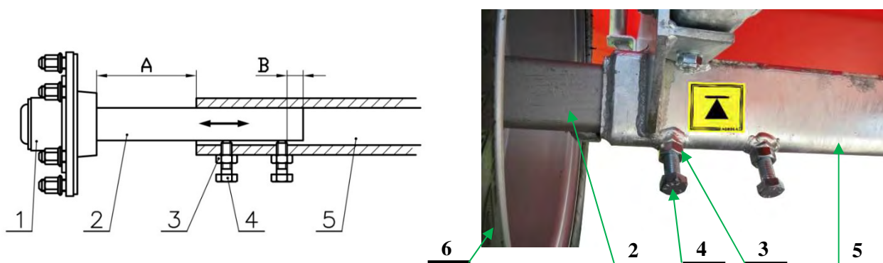
Rys. 39. Schemat regulacji rozstawu kół opryskiwacza
