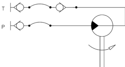
Rys. 44. Schemat hydrauliczny podłączenie silnika hydraulicznego pompy wirowej mieszadeł.
