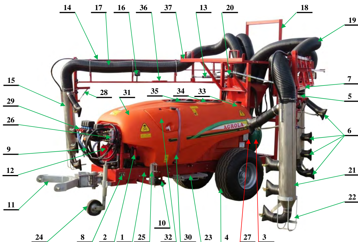
Rys. 5. Widok z boku opryskiwacza sadowniczego przyczepianego AGROLA HST do upraw rzędowych
