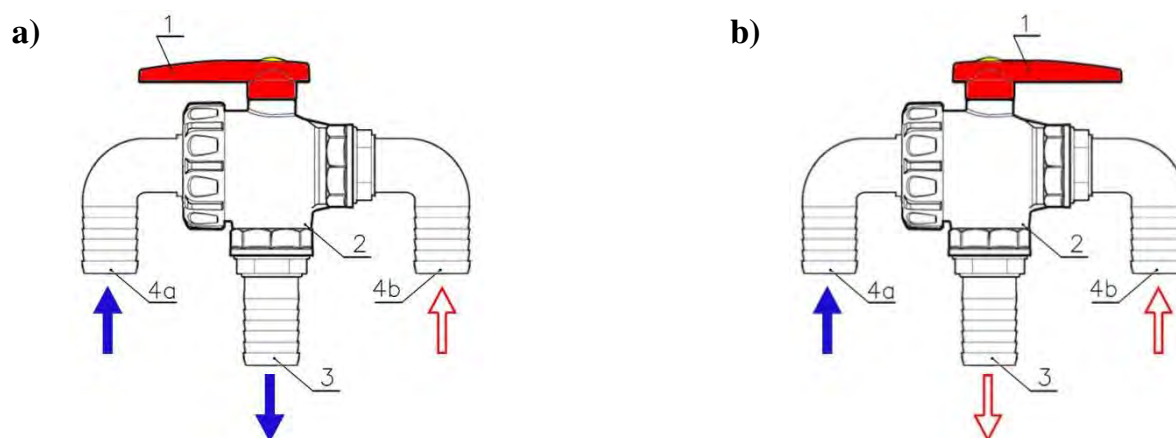
Rys. 13. Zawór trójdrożny - schemat
