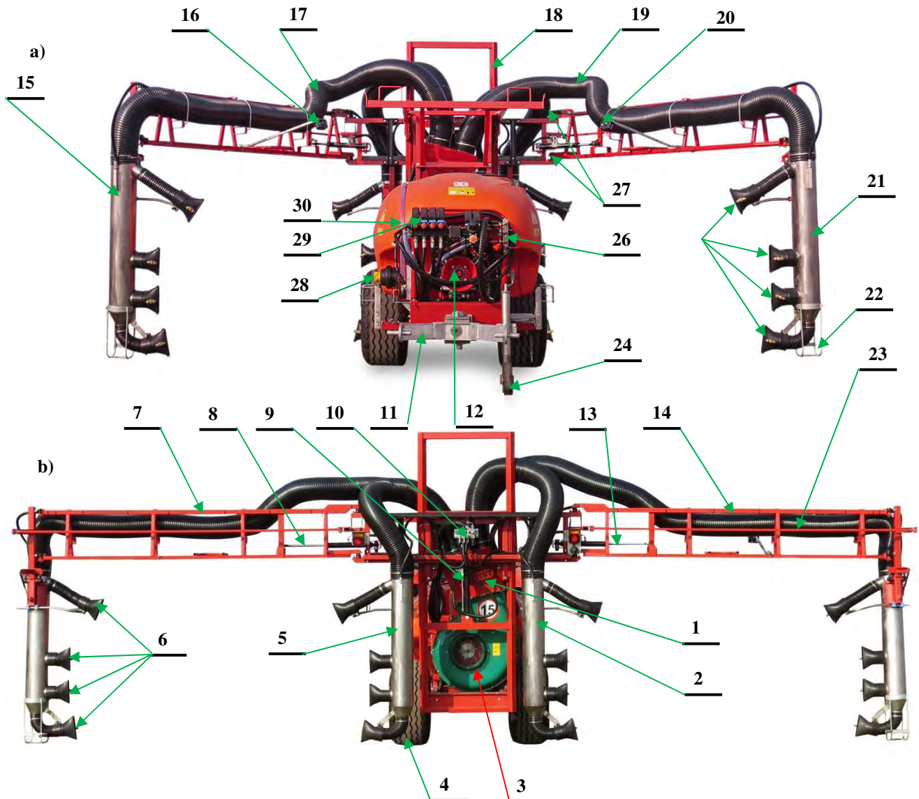
Rys. 4. Widok opryskiwacza sadowniczego przyczepianego AGROLA HST do upraw rzędowych
