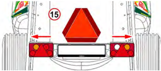
Rys. 46. Ustawienie tylnej instalacji świateł drogowych w pozycji na czas przejazdów drogowych
