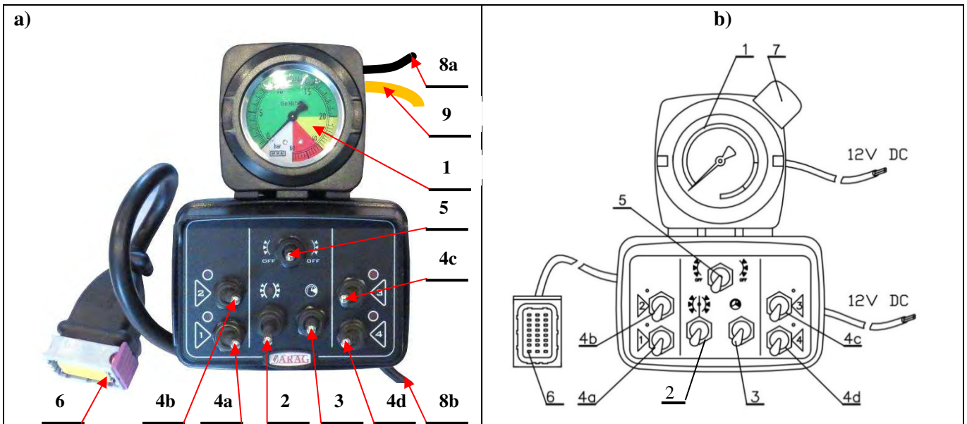
Rys. 23. Pulpit sterowniczy ARAG
