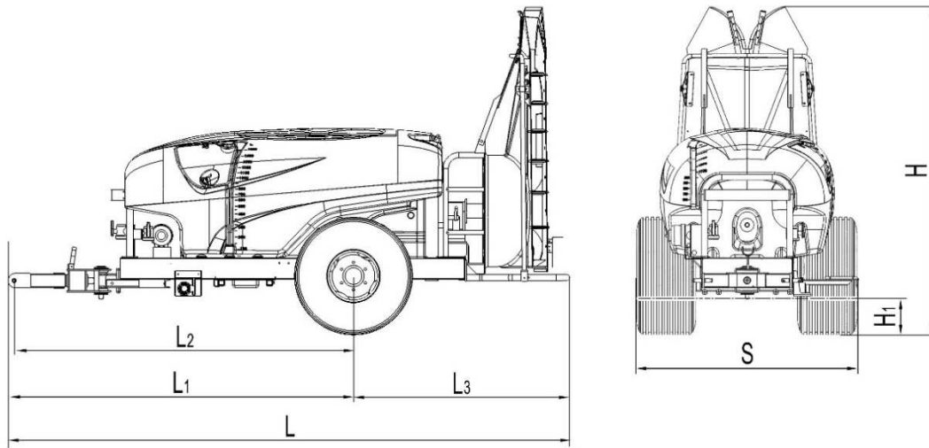
Rys. 6. Schemat wymiarów opryskiwacza
