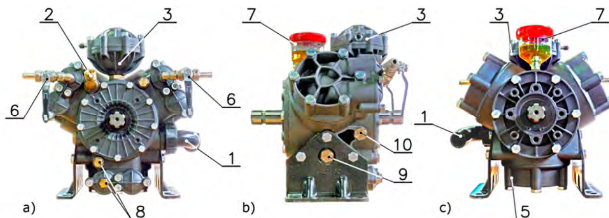
Rys. 10. Pompa AR 1203. Widok po zdjęciu osłony stożkowej
