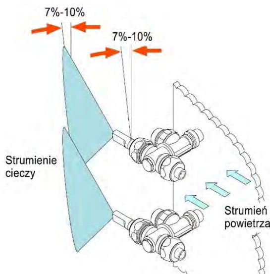
Rys. 34. Schemat montażu rozpylaczy płaskostrumieniowych
