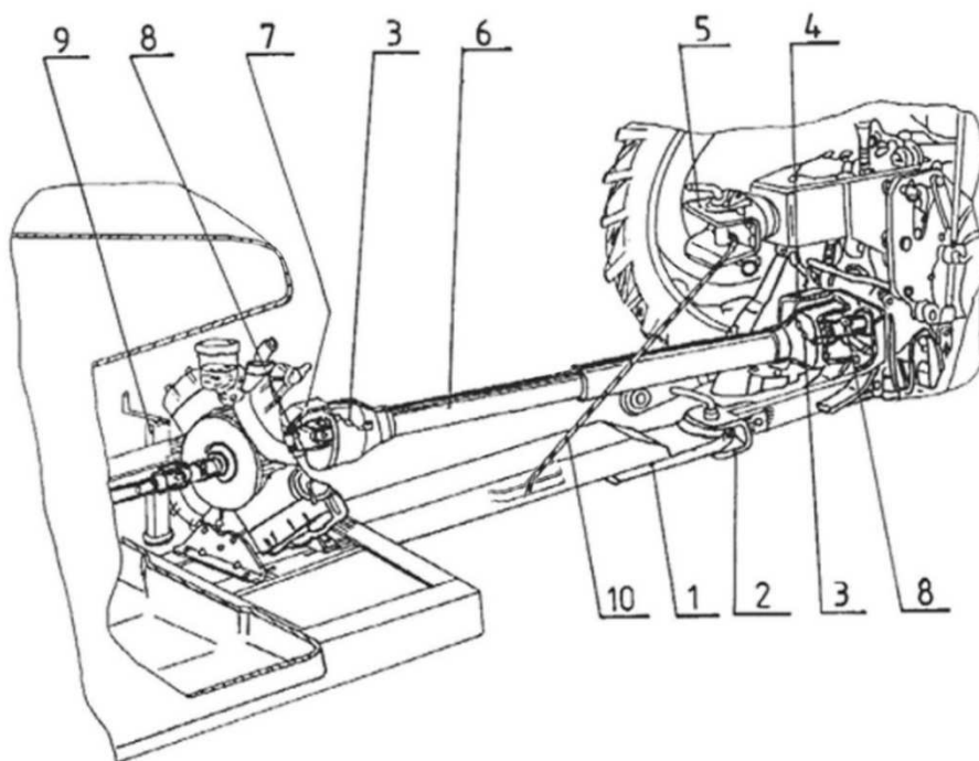
Rys. 51. Agregowanie opryskiwacza z ciągnikiem
