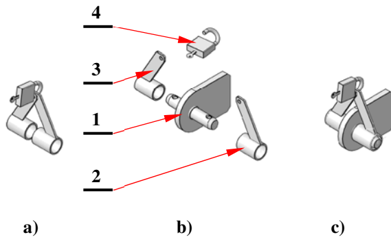
Rys. 50. Zabezpieczenie antykradzieżowe montowane na dyszlu skrętnym v2-2N (CSD-A1.00.00)
