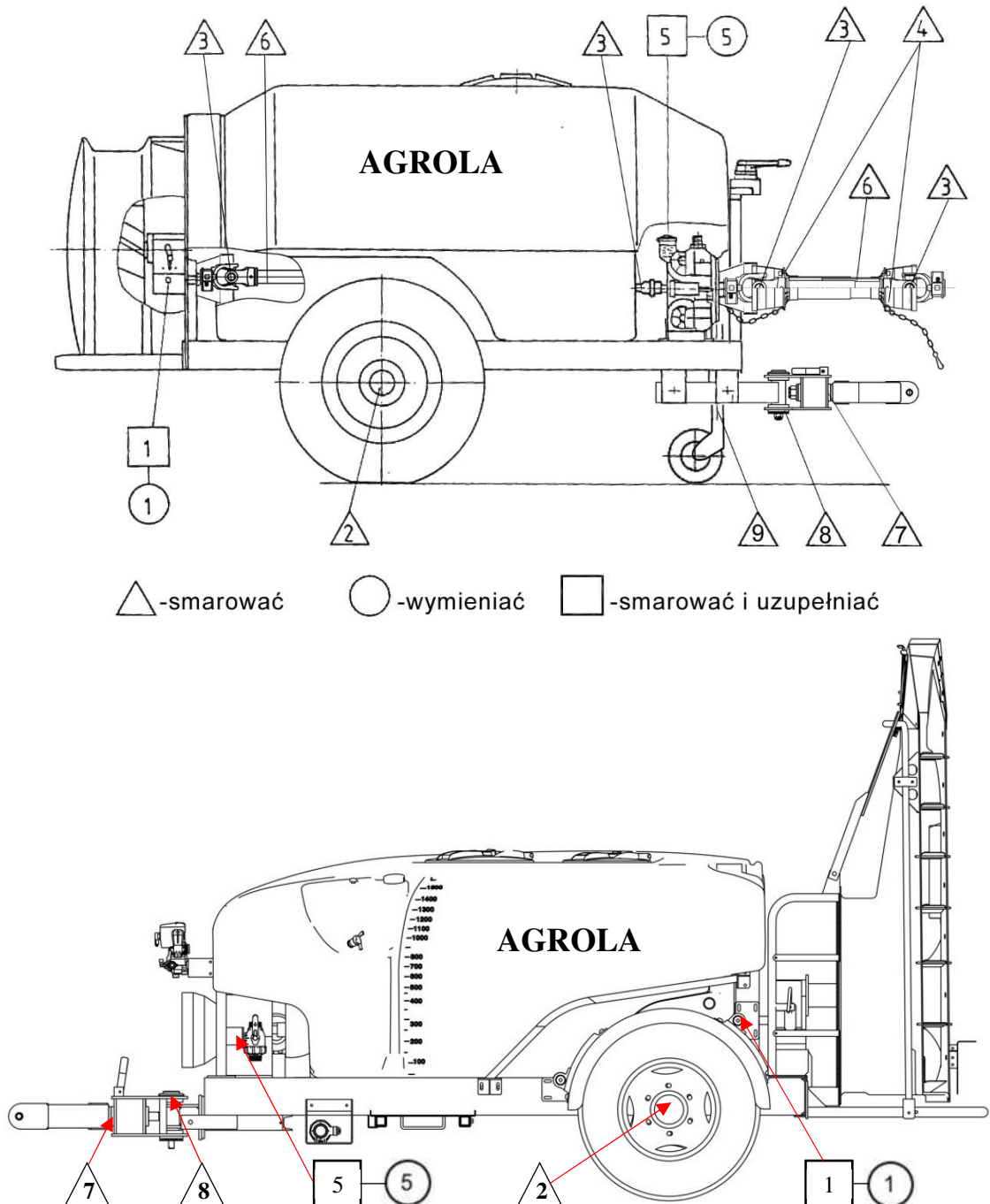
Rys. 52. Rozmieszczenie punktów smarowania
