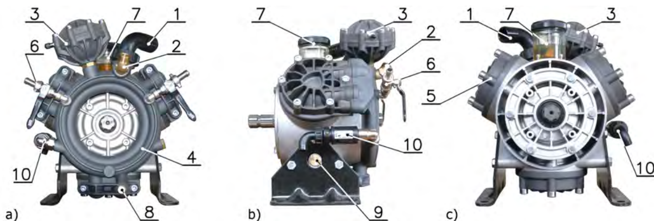
Rys. 11. Pompa BHA 130; BHA150. Widok po zdjęciu osłony stożkowej
