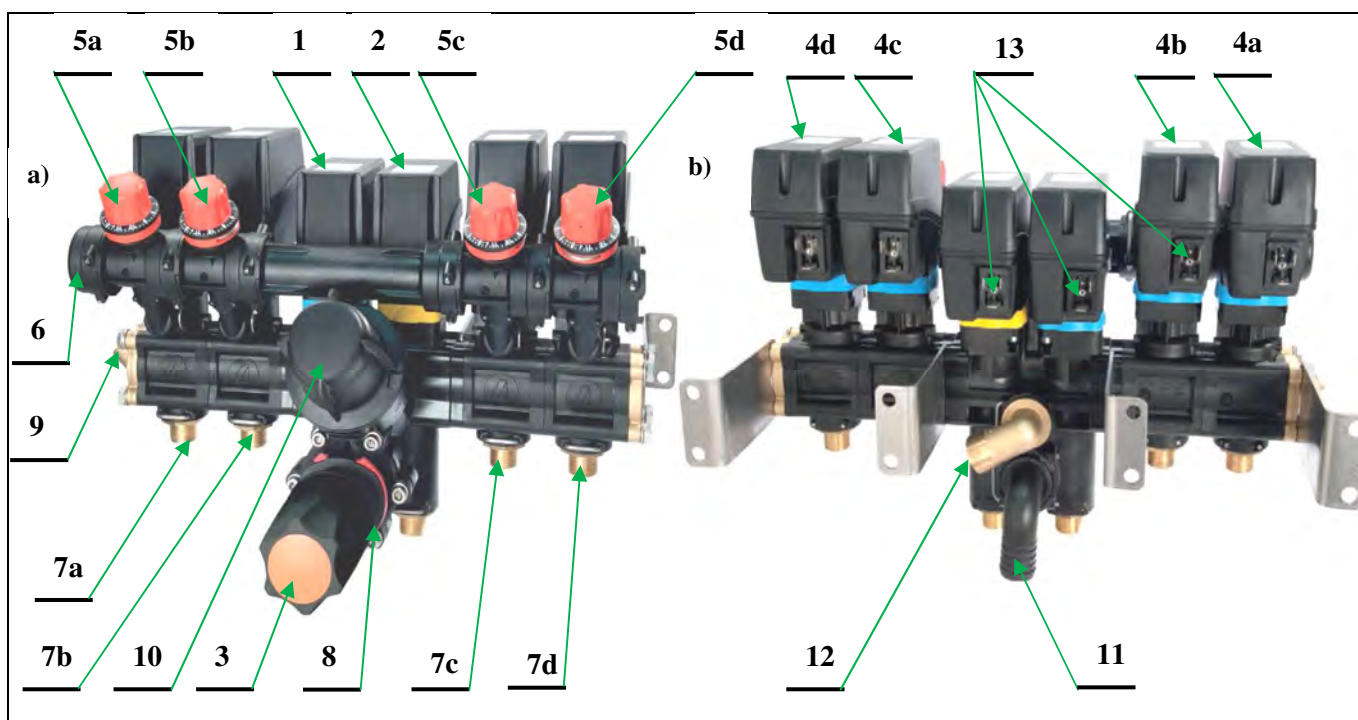
Rys. 21. Elektrozwór ARAG sterujący cieczą do współpracy z manualnym pulpitem sterującym:
