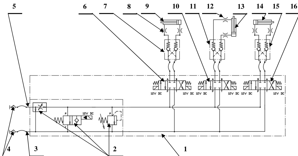
Rys. 7. Schemat układu hydraulicznego opryskiwacza do upraw rzędowych AGROLA HST
