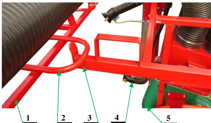
Rys. 32. Uchwyt podpierający zespół opryskowy podczas transportu
