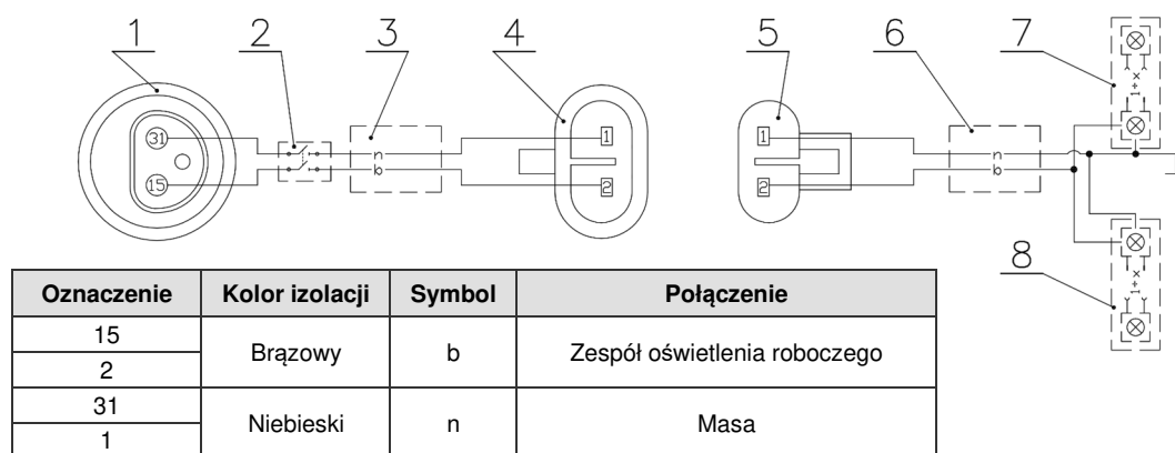
Rys. 41. Schemat instalacji elektrycznej oświetlenia roboczego
