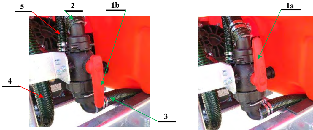
Rys. 14. Zawór trójdrożny - widok
