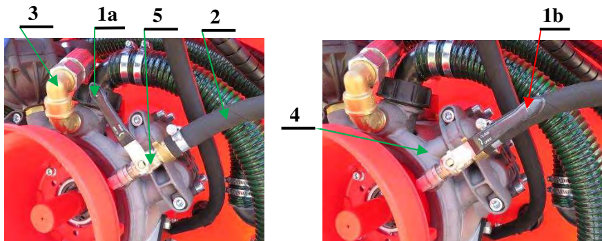
Rys. 15. Zawór zasilający listwę zaworów (kolektor)
