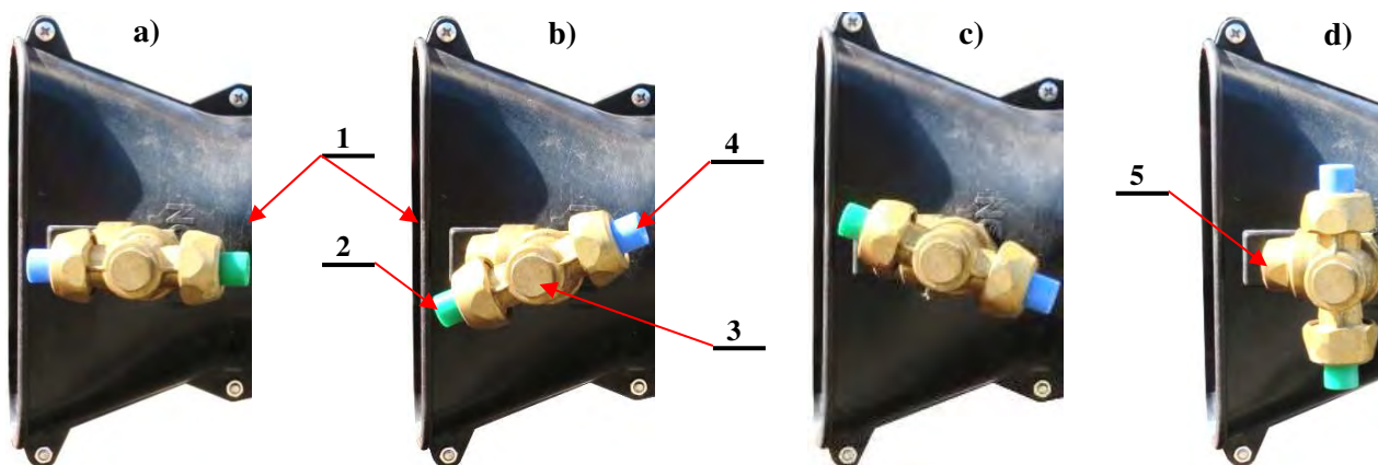
Rys. 30. Dyfuzor z oprawą rozpylaczy
