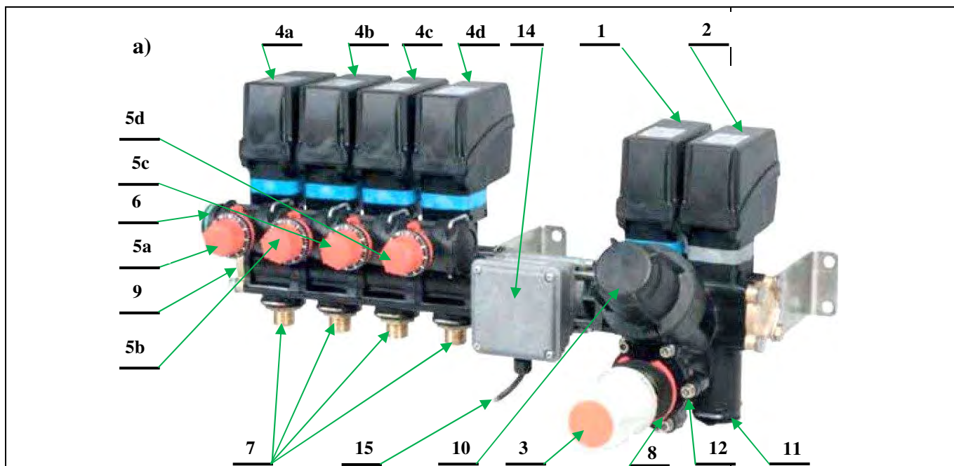
Rys. 24. Elektrozwór ARAG sterujący cieczą do współpracy z komputerem Bravo 350
