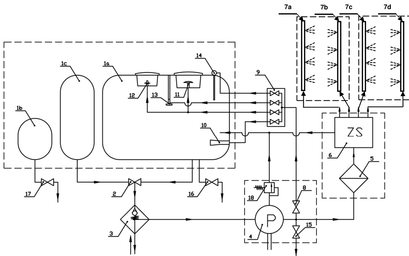
Rys. 3. Schemat działania i obiegu cieczy ze zbiornikiem 3-częściowym.
